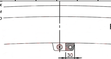
Рис. 2 (схема подрезки бампера).
